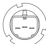
H6W - BAX9s
